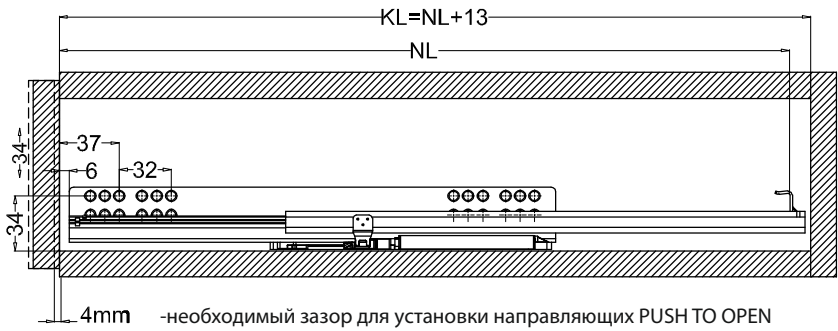
ВНУТРЕННИЙ МОНТАЖ
