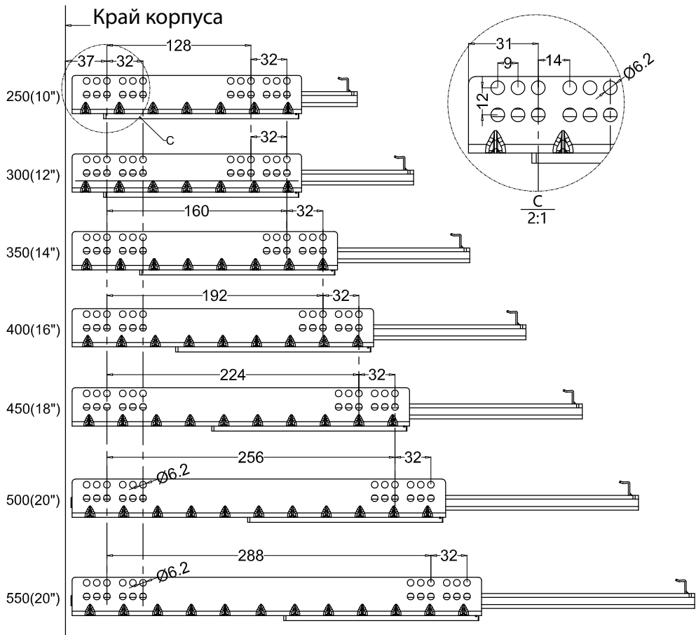
РАСПОЛОЖЕНИЕ КРЕПЕЖНЫХ ОТВЕРСТИЙ
