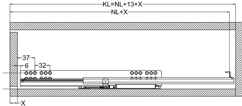
ВНУТРЕННИЙ МОНТАЖ
