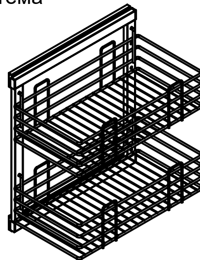
2-х ур. корзина Габаритные размеры (ШхГхВ) 285x475x515
