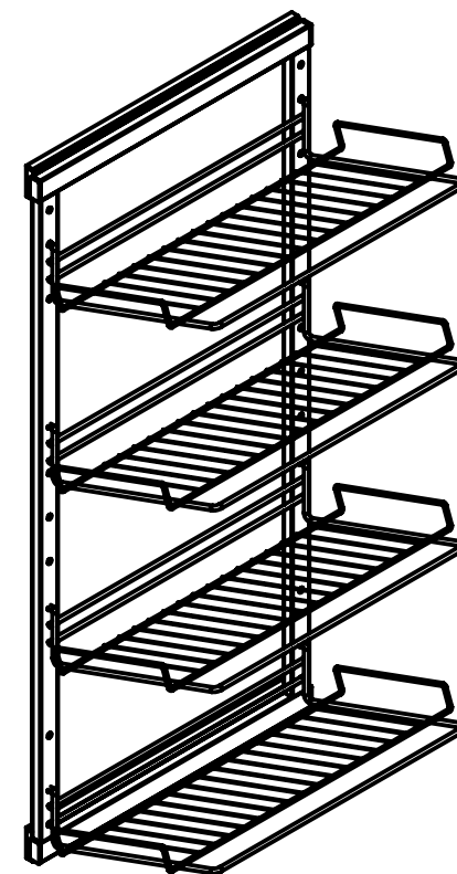
4-х ур. обувница Габаритные размеры (ШхГхВ) 315x480x1015
