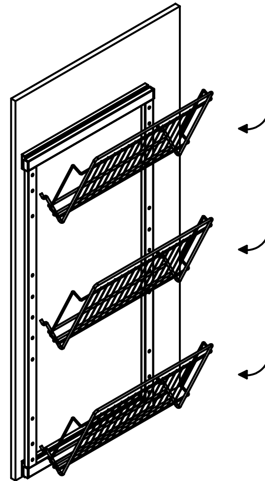
4. Установка корзин на раму
