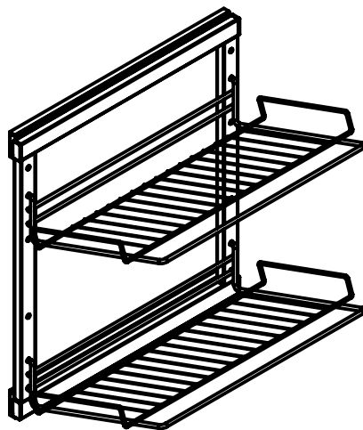
2-х ур.обувница Габаритные размеры (ШхГхВ) 315x480x515
